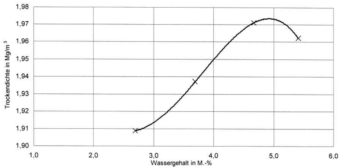
Proctorkurve des Baustoffgemisches 0/32 (FSS)
